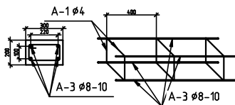
Фрагмент каркаса монолитного пояса
